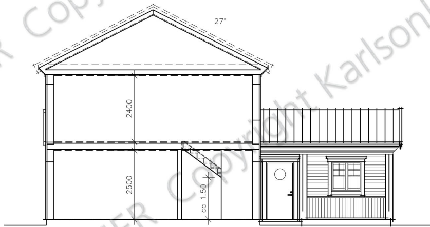
SEKTION A
